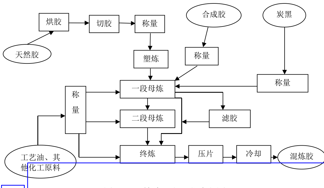
图 2.2-3 炼胶工段工艺流程图
