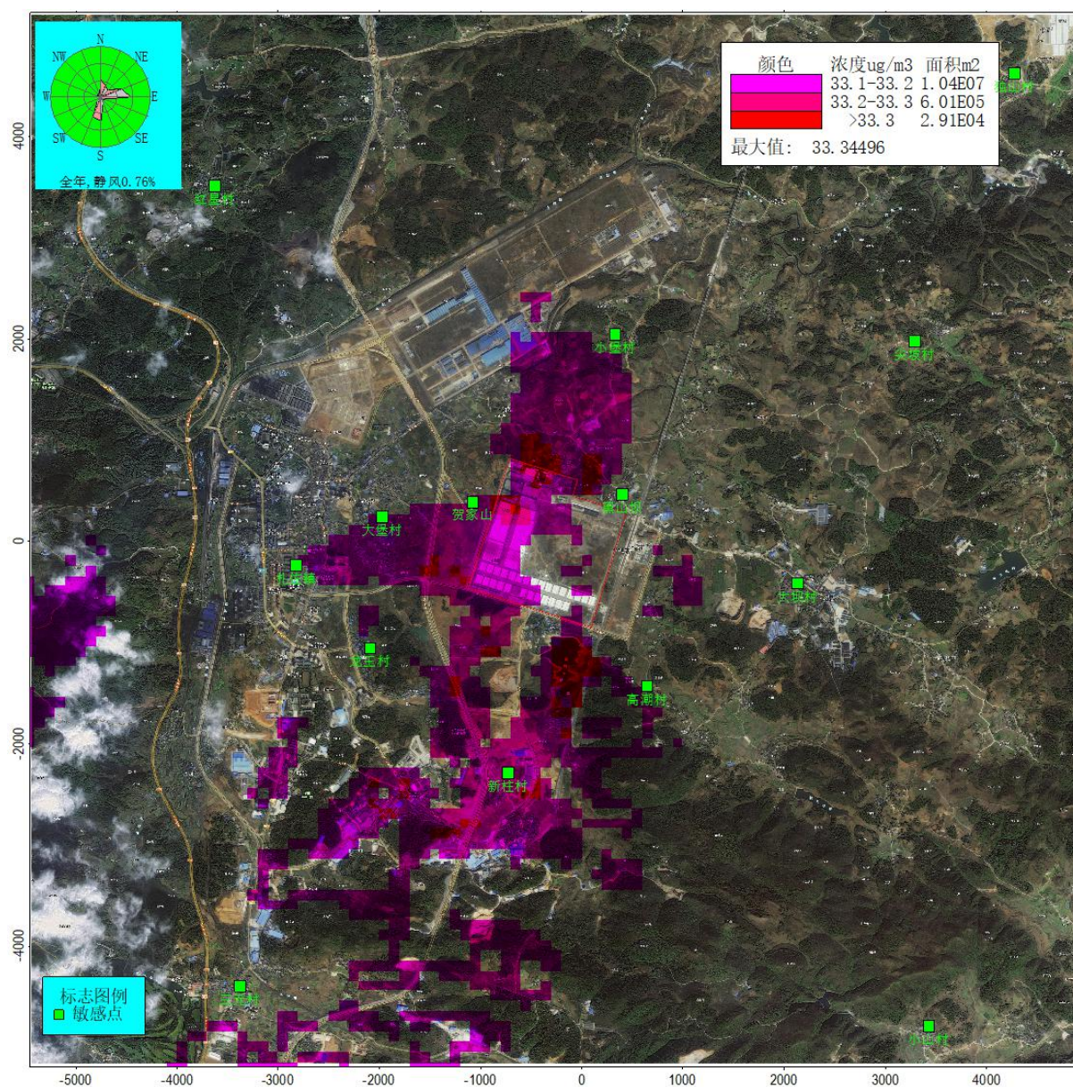
图 4.3-8 叠加后网格点 \text{PM}_{10} 年平均质量浓度分布图
